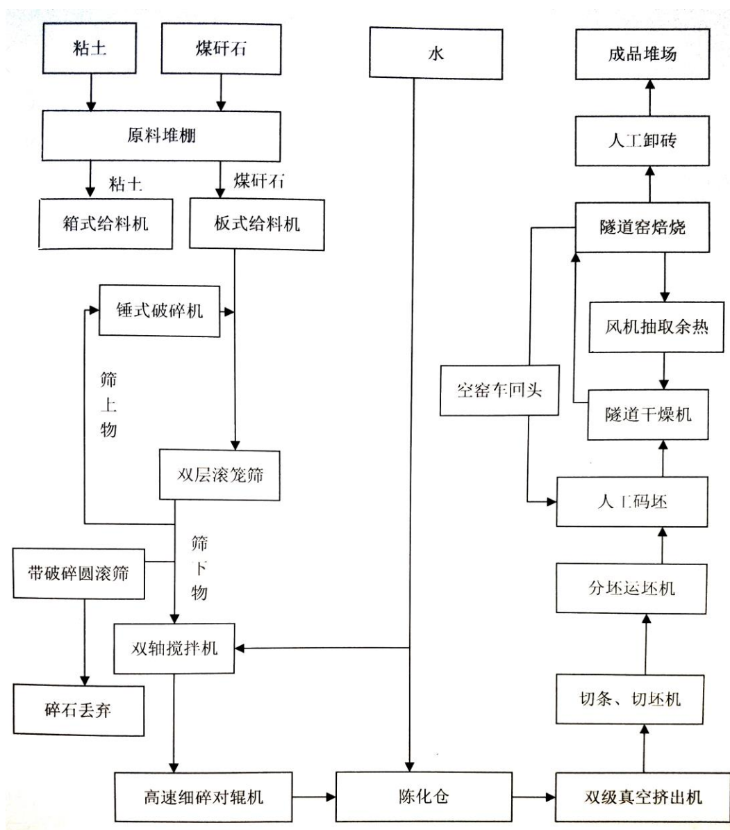
图 5-1 工艺流程图
