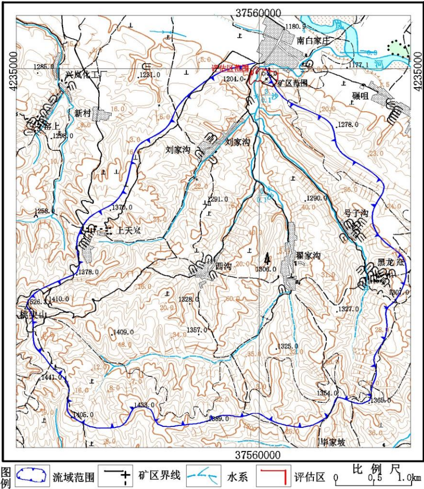
图 8-4 沟谷流域图
