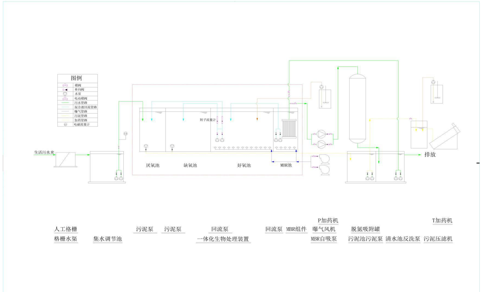
工艺流程图
